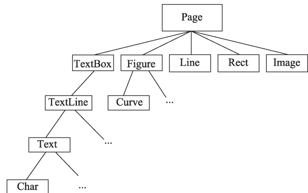
图 2 PDFminer 解析 PDF 的物理结构树
