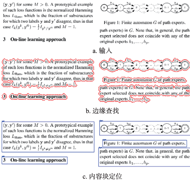
图 1 利用机器视觉处理学术论文的过程
